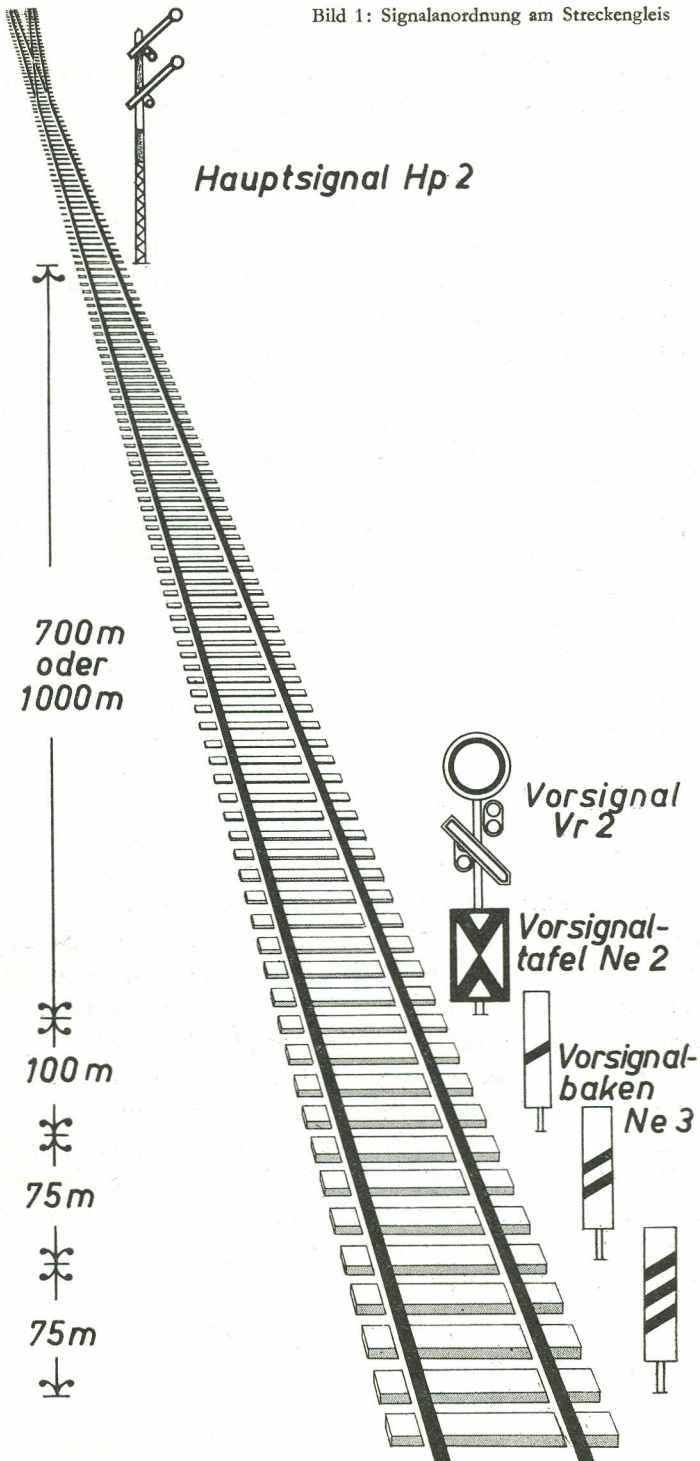
Bild 1: Signalanordnung am Streckengleis
