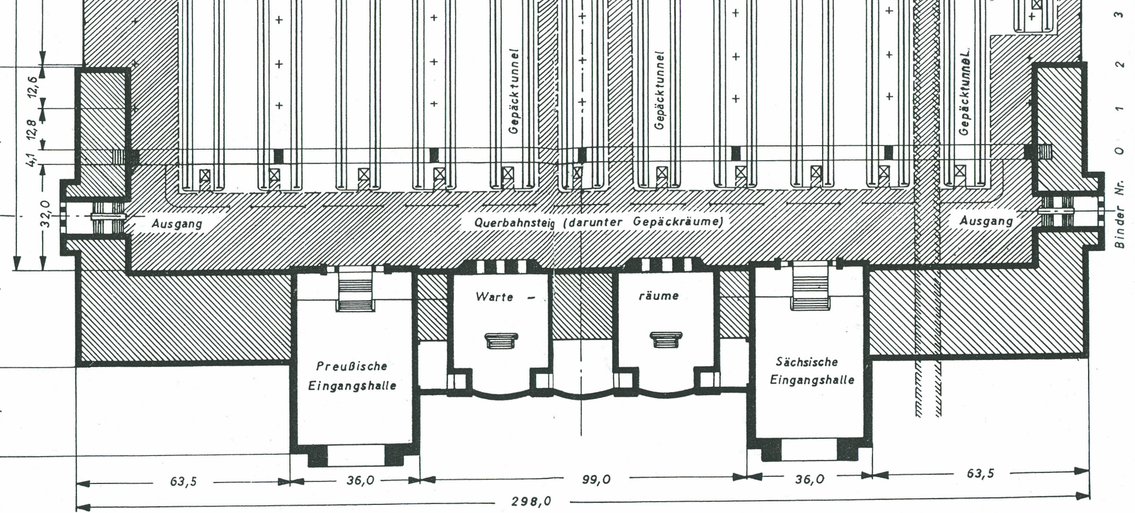
17 Übersicht Grundriß der Bahnsteige und des Empfangsgebäudes
