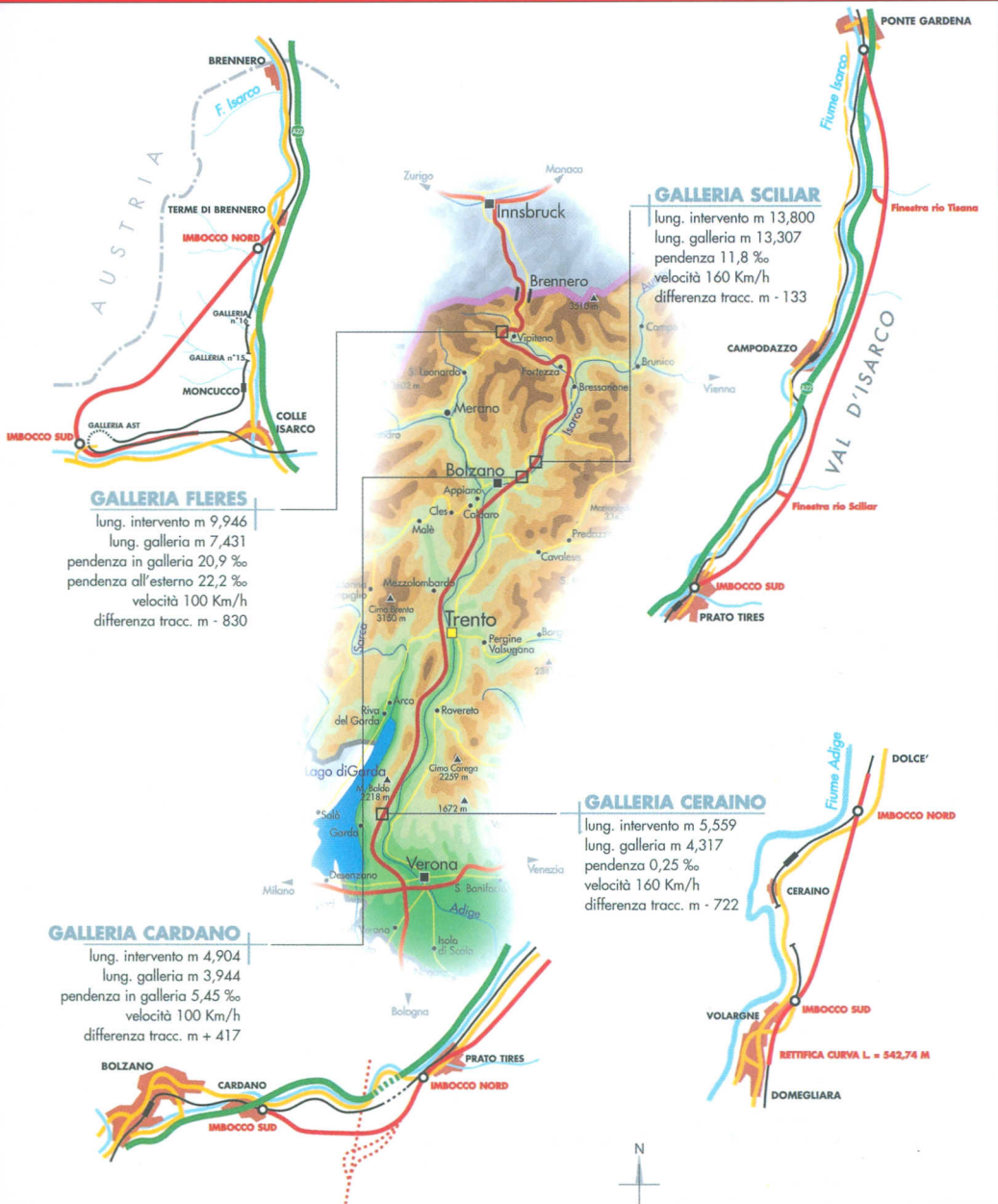
Darstellung der 1994 bis 1999 in Betrieb genommenen Tunnelvarianten zwischen Brenner und Verona (Flerés/Pflersch, Sciliar/Schlern, Cardano/Kardaun und Ceraino in der Berner Klause knapp vor Verona)
